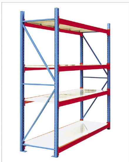
DC-50型 (均载450KG/层) 规格: 长2000mm宽600mm高2000mm
