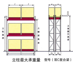
立柱最大承重量 型号 (双C复合梁)
