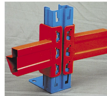
DC-70型(均载450~1000KG/层) 规格:长2000~2500mm宽(600~900mm)x高(2000~4000mm)
