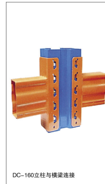
DC-160立柱与横梁连接
