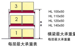
每层最大承重量
