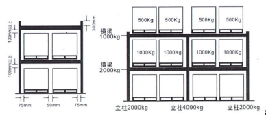
重型托盘货架(横梁式货架)堆放尺寸图
